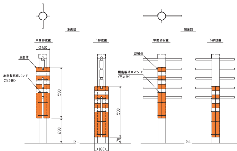
PW-L-WR-2 設置例
